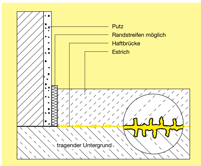
Bild 4: Verbundestrich [4]
