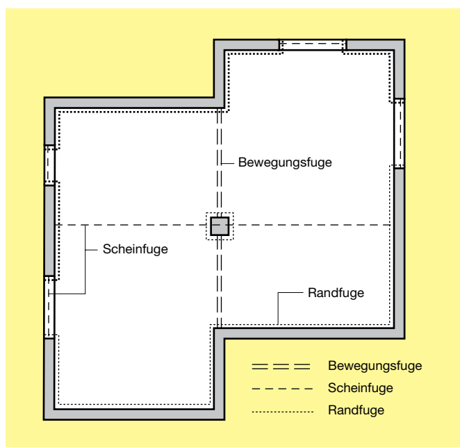
Bild 13: Beispiel eines Fugenplans [4]
